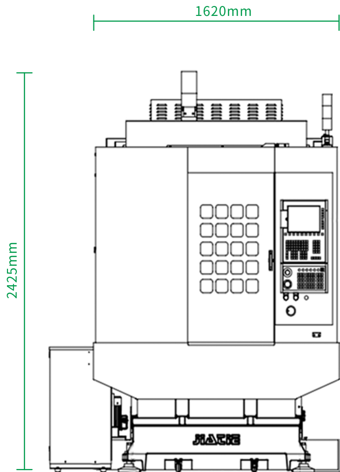
前视图
