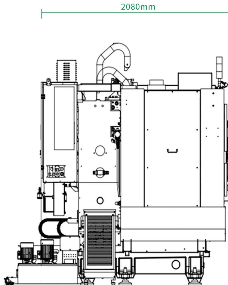
侧视图
